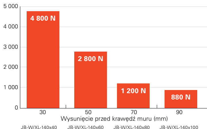
Nośność F_{Rk} [N]
