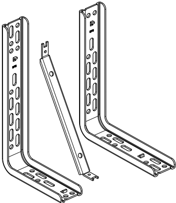
JB-A / JB-AS 150×280 mm 205×240 mm 190 mm
