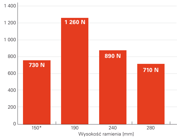
Nośność F_{Rk} [N]
