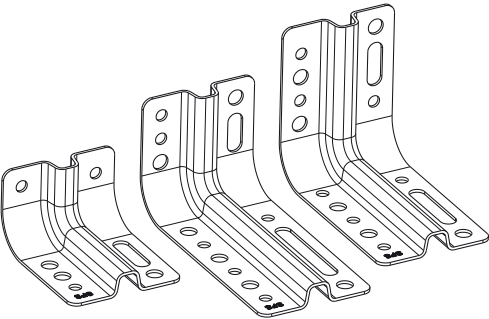
JB-W 70×40 mm 100×60 mm 120×80 mm
